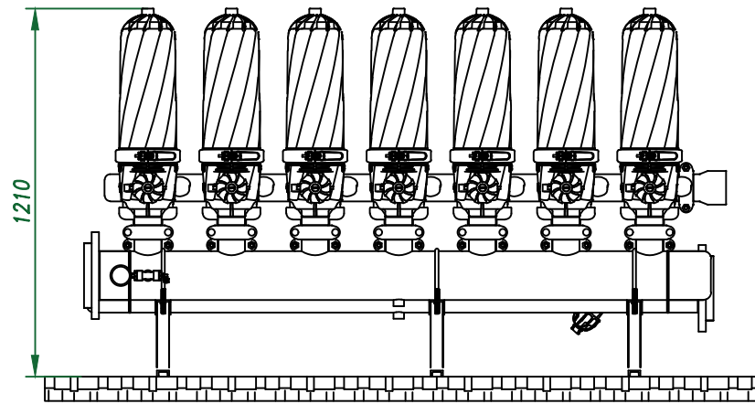
Вид спереди
