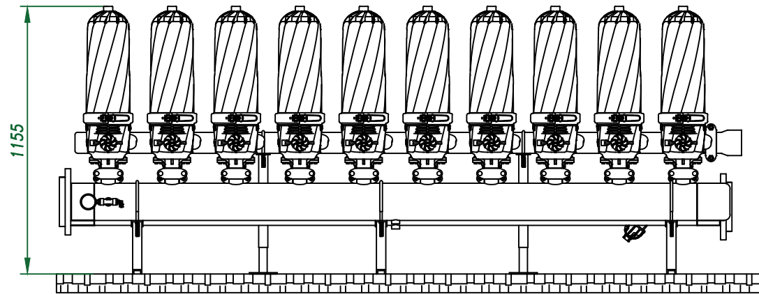
Вид спереди
