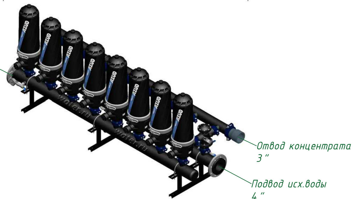
Изометрия
