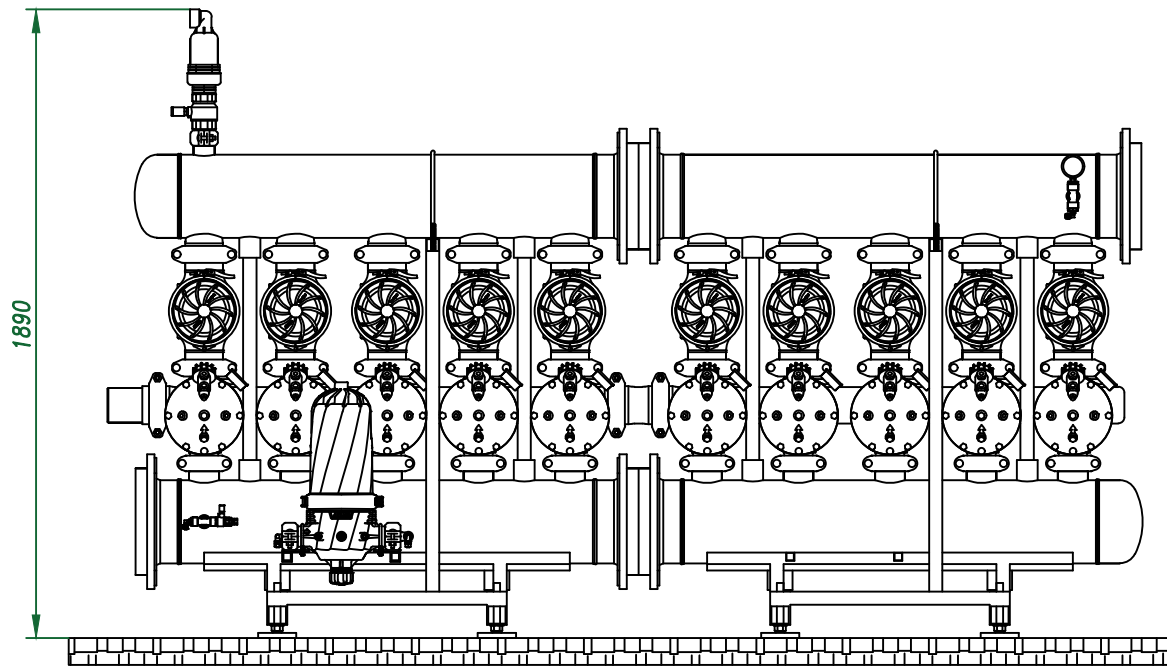
Вид спереди
